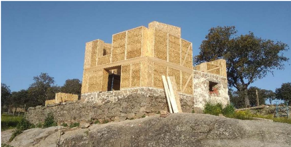
Imagen superior derecha: Entramado prefabricado de madera y corcho granulado. Imagen superior izquierda: Entramado prefabricado de madera y fibra de madera. Imagen superior: entramados prefabricados de madera y paja para rehabilitación-ampliación de construcción existente.
